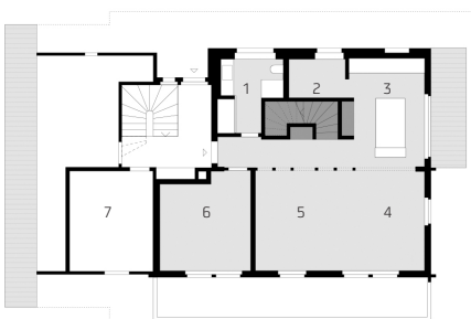
Erdgeschoss
